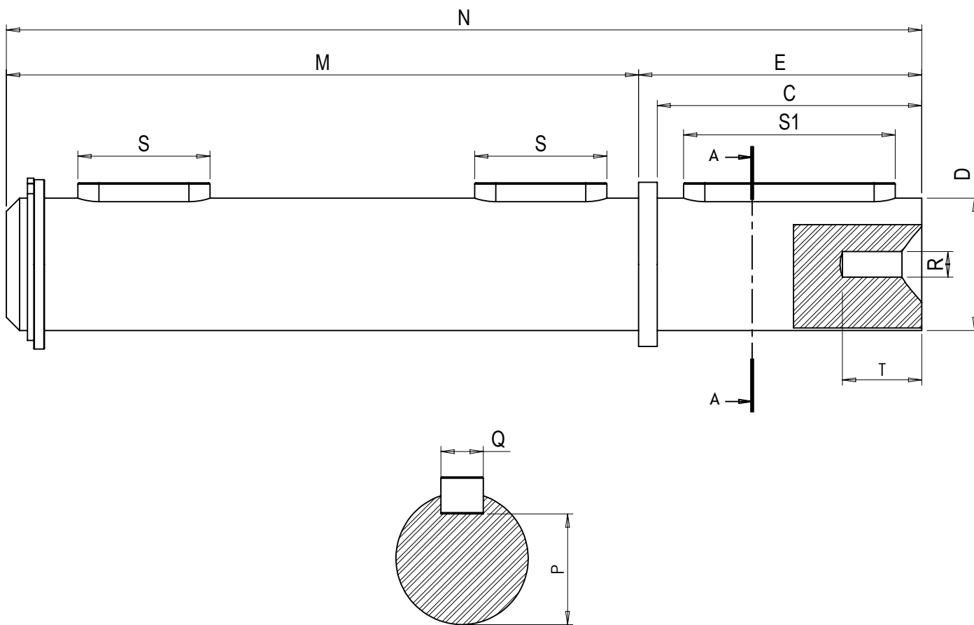
SECCIÓN A-A ESCALA 1 : 1
