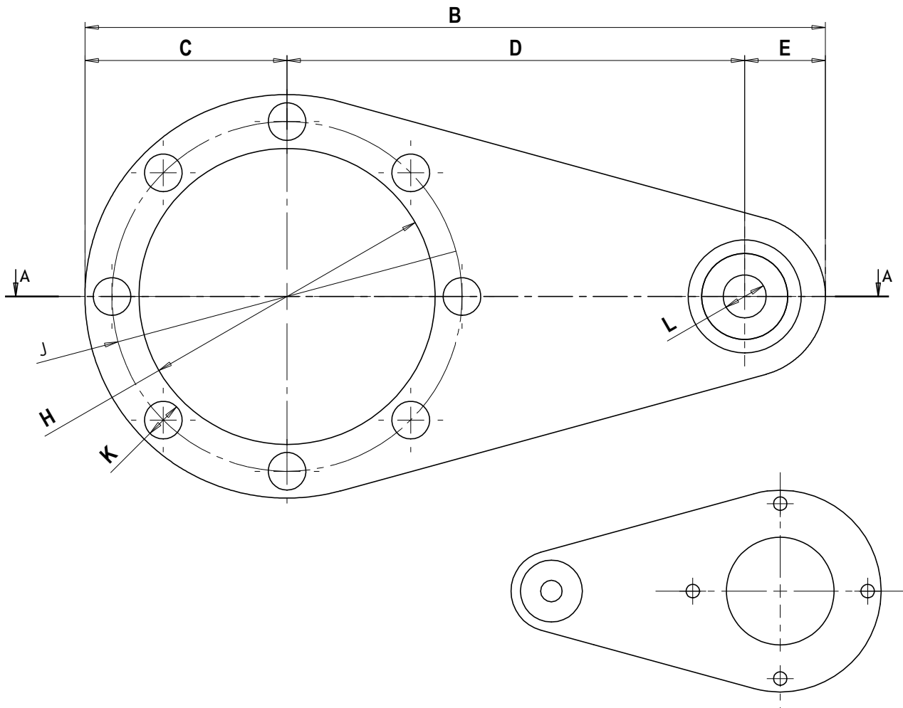
POSICIÓN TALADROS KM-30
