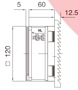
风扇及过滤器 Fan and filter JL9803.230
