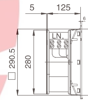
风扇及过滤器 Fan and filter JL906.230
