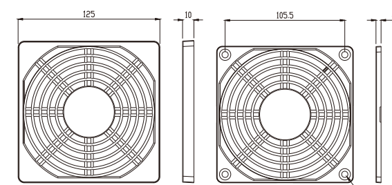
JL-12 For 120mm Fan
