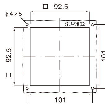
安装剖面 Mounting profile JL9802
