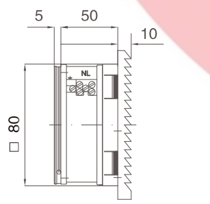
风扇及过滤器 Fan and filter JL9801.230
