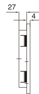
出口过滤器 Outlet filter JL902.200
