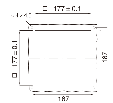
安装剖面 Mounting profile JL300
