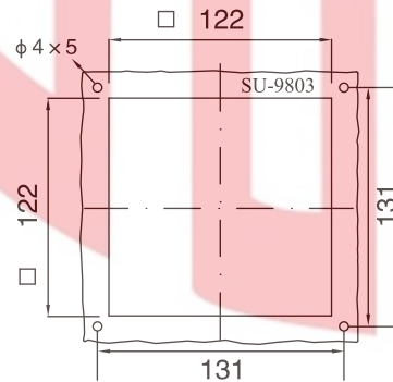
安装剖面 Mounting profile JL9803
