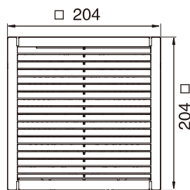
风扇及过滤器 Fan and filter JL903
