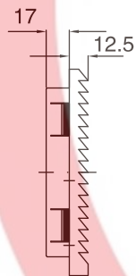
出口过滤器 Outlet filter JL600.300
