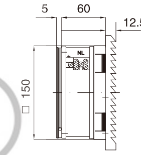
风扇及过滤器 Fan and filter JL9804.230
