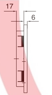
出口过滤器 Outlet filter JL905.200
