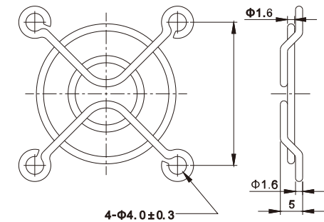
JL-06 For 60mm Fan
