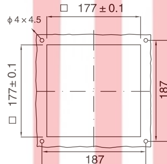
安装剖面 Mounting profile JL903
