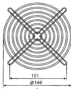
JL-150 FOR 150MM FAN
