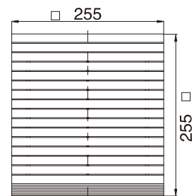
风扇及过滤器 Fan and filter JL9805
