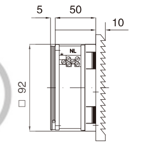
风扇及过滤器 Fan and filter JL9802.230
