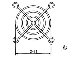
JL-50 FOR 50MM FAN
