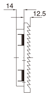
出口过滤器 Outlet filter JL9805.200
