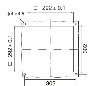
安装剖面 Mounting profile JL906
