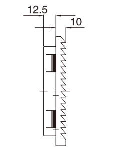
出口过滤器 Outlet filter JL9801.200
