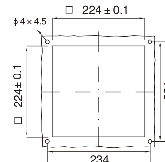
安装剖面 Mounting profile JL904
