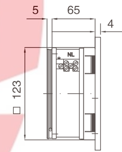
风扇及过滤器 Fan and filter JL902.230
