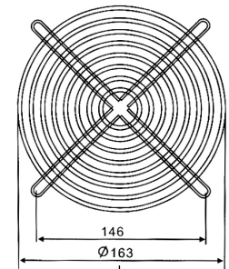
JL-170 FOR 170MM FAN
