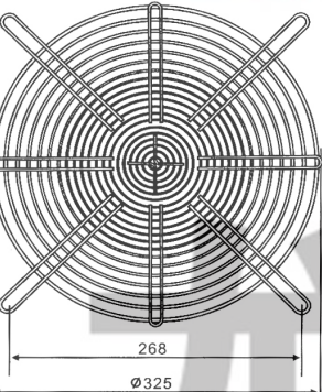
JL-300 FOR 300MM FAN
