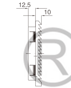
出口过滤器 Outlet filter JL9802.200
