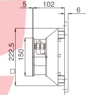
风扇及过滤器 Fan and filter JL904.230
