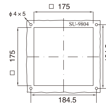
安装剖面 Mounting profile JL9804
