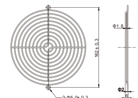
JL-15 For 150mm Fan
