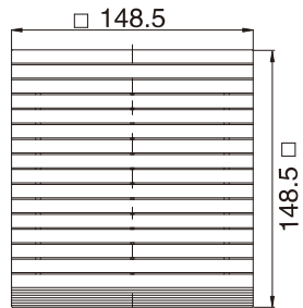
风扇及过滤器 Fan and filter JL9803
