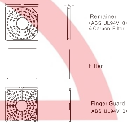
JL-06 For 60mm Fan
