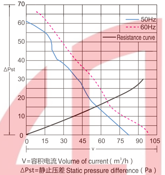
出口过滤器 Outlet filter JL200.300
