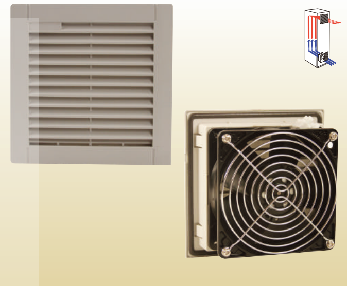
出口过滤器 Outlet filter JL902.200
