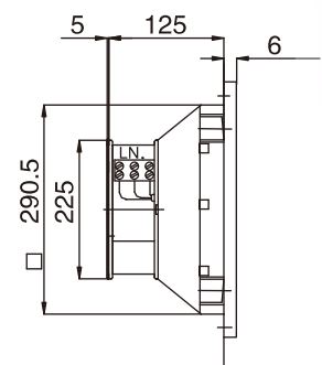
风扇及过滤器 Fan and filter JL905.230
