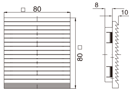
风扇及过滤器 Fan and filter JL9800 出口过滤器 Outlet filter JL9800.200
