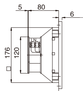
风扇及过滤器 Fan and filter JL903.230
