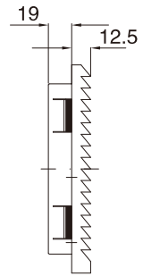
出口过滤器 Outlet filter JL9803.200
