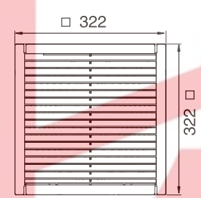
风扇及过滤器 Fan and filter JL906
