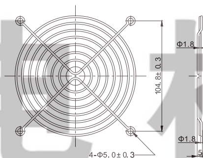
JL-12 For 120mm Fan
