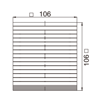
风扇及过滤器 Fan and filter JL9801
