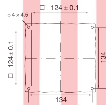
安装剖面 Mounting profile JL200
