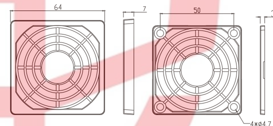
JL-09 For 92mm Fan
