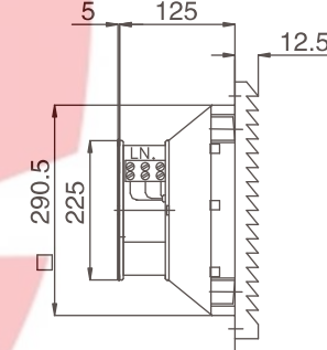
风扇及过滤器 Fan and filter JL500.230
