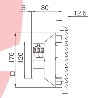
风扇及过滤器 Fan and filter JL300.230
