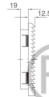
出口过滤器 Outlet filter JL9804.200
