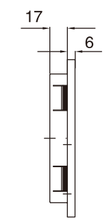
出口过滤器 Outlet filter JL906.200
