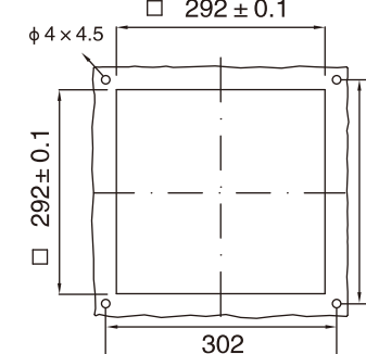
安装剖面 Mounting profile JL500
