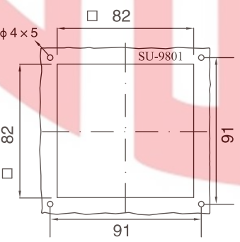
安装剖面 Mounting profile JL9801
