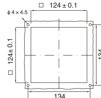
安装剖面 Mounting profile JL902
