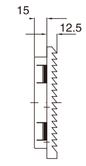
出口过滤器 Outlet filter JL300.300
