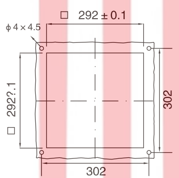
安装剖面 Mounting profile JL905
