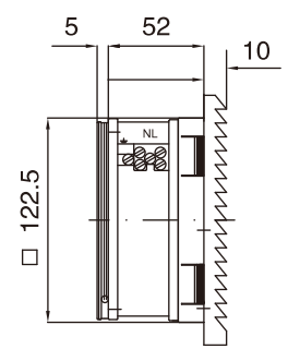
风扇及过滤器 Fan and filter JL200.230
