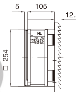
风扇及过滤器 Fan and filter JL9806
