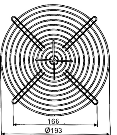
JL-200 FOR 200MM FAN
