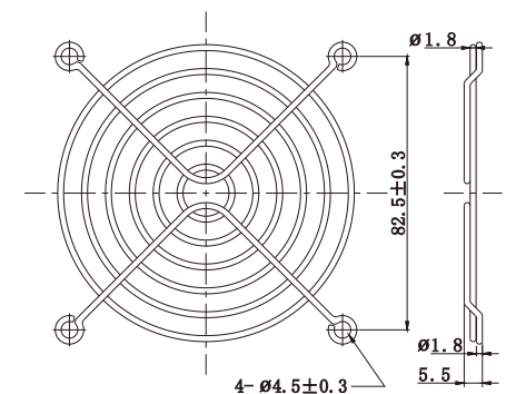
JL-09 For 92mm Fan
