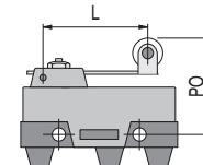
M3L21 - Palanca con Rodillo y Punto de Operación Regulable
