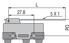
M3G - Palanca Larga M3H - Palanca Larga
