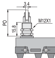
M3S2 - Botón p/Paineil con Rodillo Transversal
