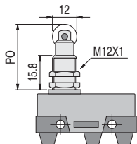
M3S1 - Botón para Paineil con Rodillo
