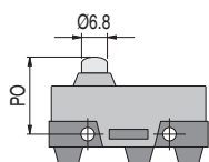
M3F - Botón Corto
