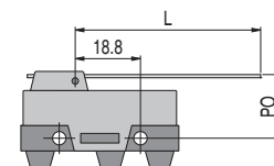
M3M - Palanca Larga con Operación Invertida
