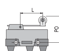
M3P - Palanca Corta con Rodillo y Operación Invertida
